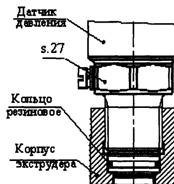
Рисунок 8 – Пример разметки монтажного гнезда и установки датчика МИДА-ДИ-12П-072
