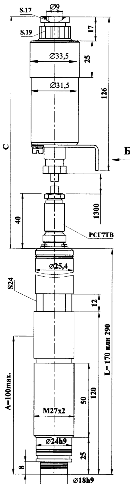
Рисунок 1 С прямым сальниковым вводом Резьба М27х2
