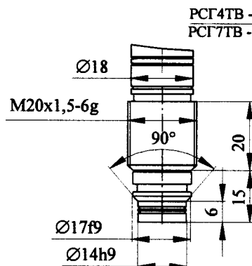
Рисунок 4 Резьба M20x1,5 Остальное см. рисунок 1.
