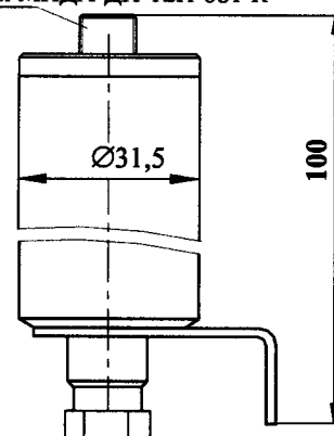
Рисунок 3 С разъемом Остальное см. рисунок 1,2. PCГ4ТВ – для МИДА-ДИ-12П-081(-В) PCГ7ТВ – для МИДА-ДИ-12П-081-К
