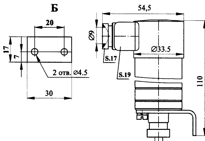
Рисунок 6 С угловым сальниковым вводом Остальное см. рисунок 1,2,3,4.
