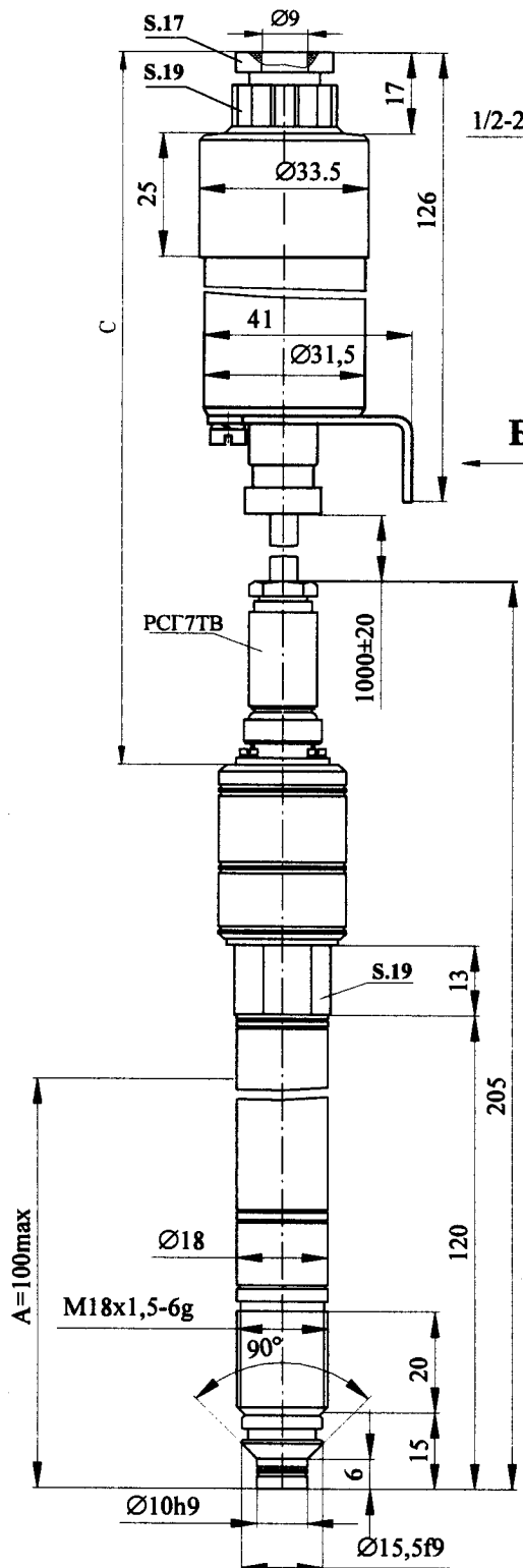
Рисунок 1 С прямым сальниковым вводом Резьба M18x1,5
