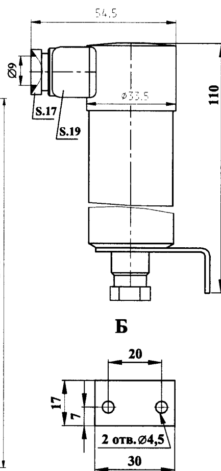
Рисунок 4 С угловым сальниковым вводом Остальное см. рисунок 1,2.
