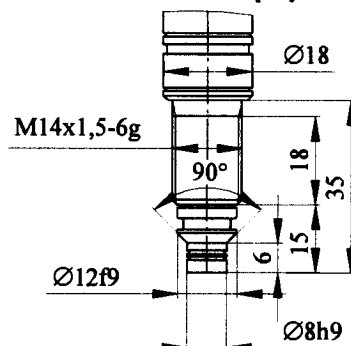
Рисунок 5 С разъемом Остальное см. рисунок 1,2,3,4.
