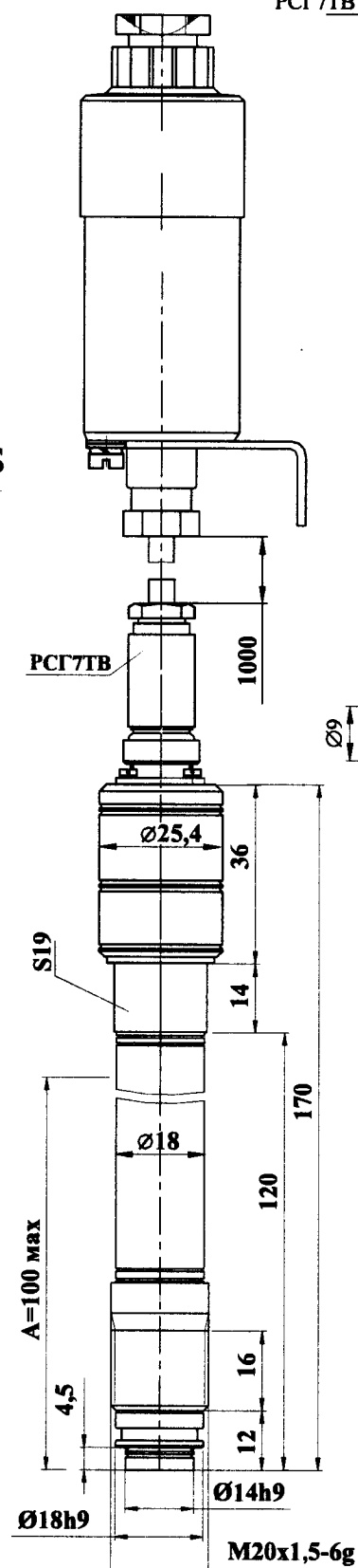
Рисунок 4 С угловым сальниковым вводом Остальное см. рисунок 1,2.
